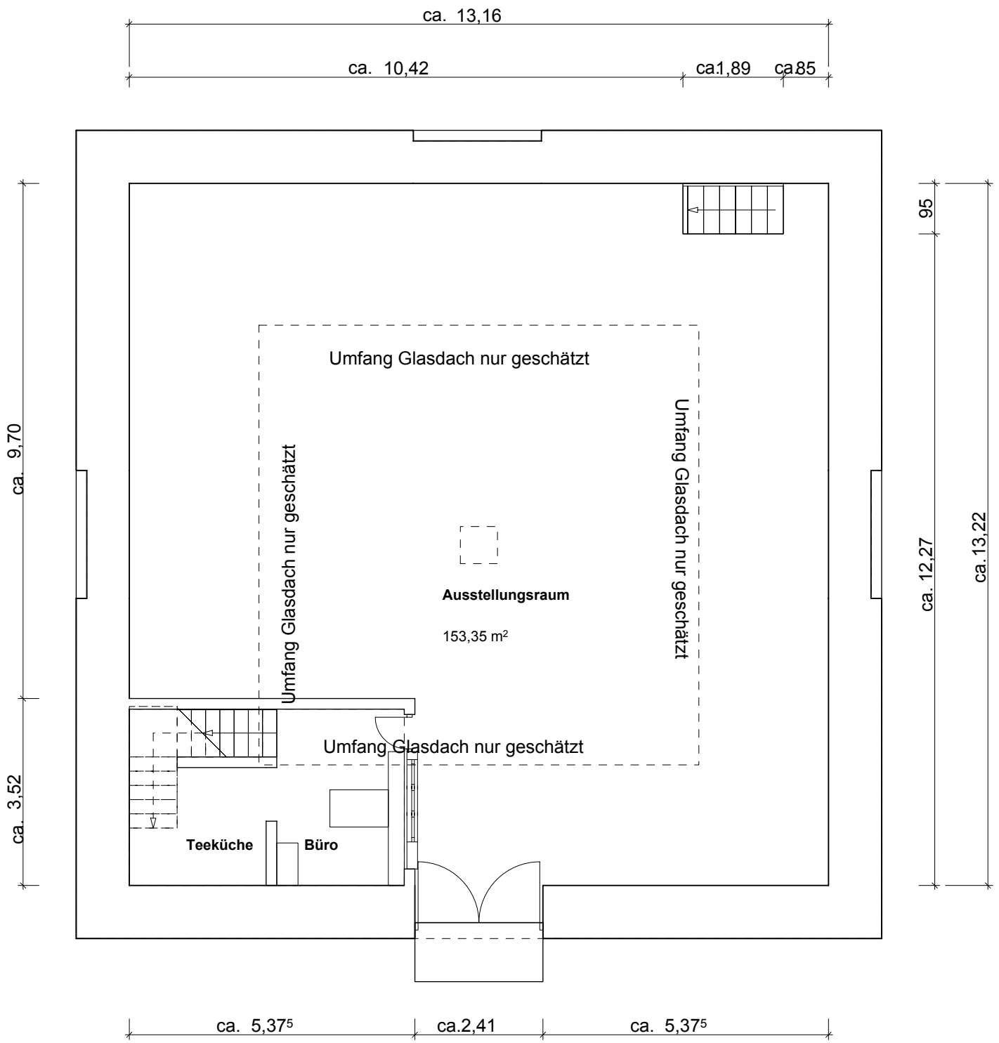
KUNSTPAVILLON Grundriss 04.11.2009
